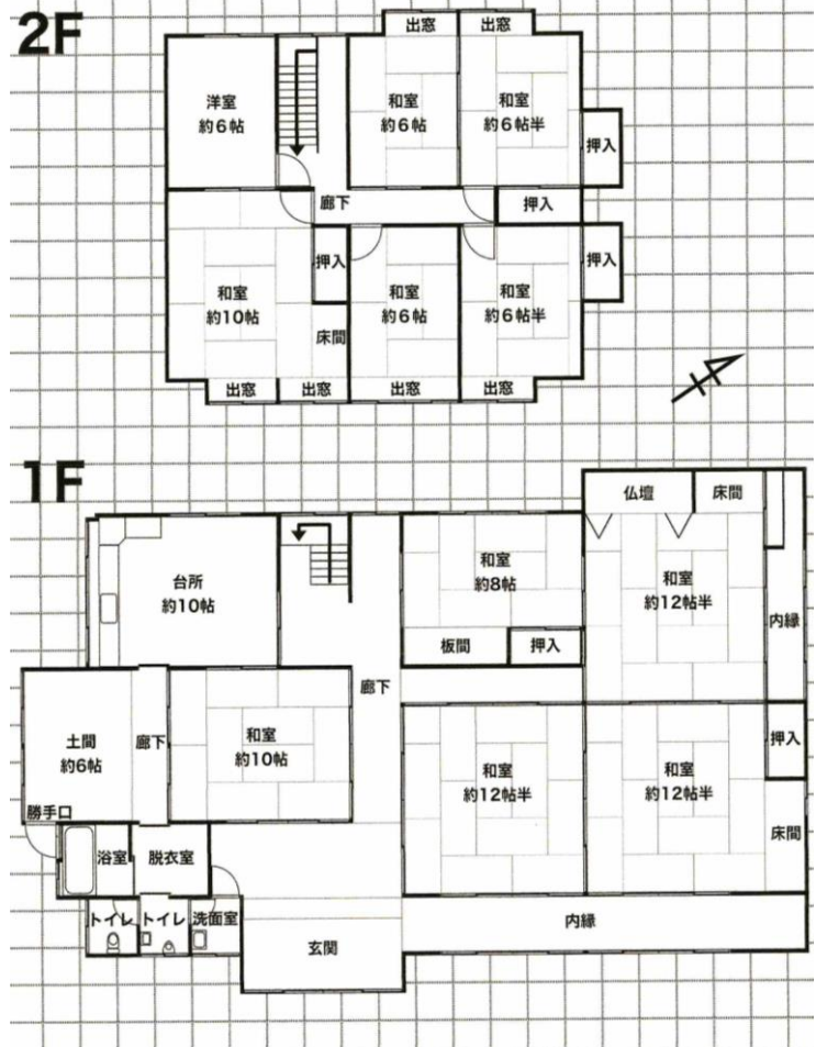
平面図
